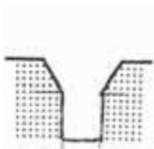
Profiel Achterstraat
