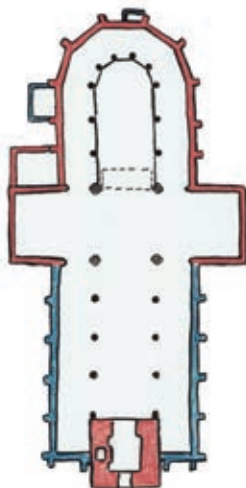
PLATTEGROND 2 1422-1516 Nieuw schip met smalle zijbeuken
